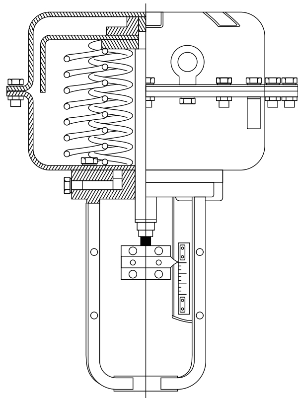
DIAPHRAGM ACTUATOR
